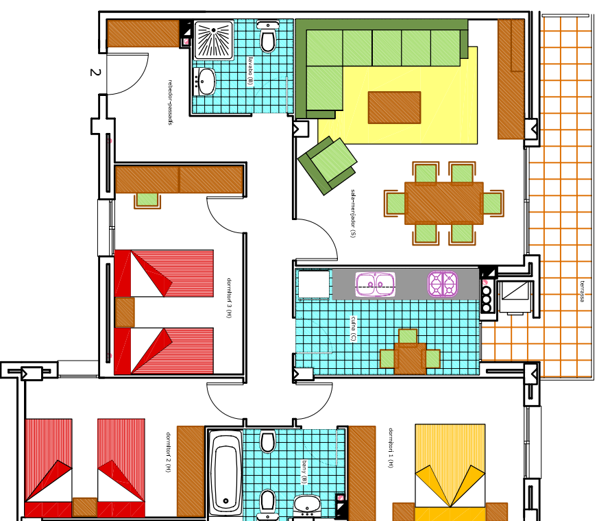
ESCALA A, PLANTA 2, PORTA 2
